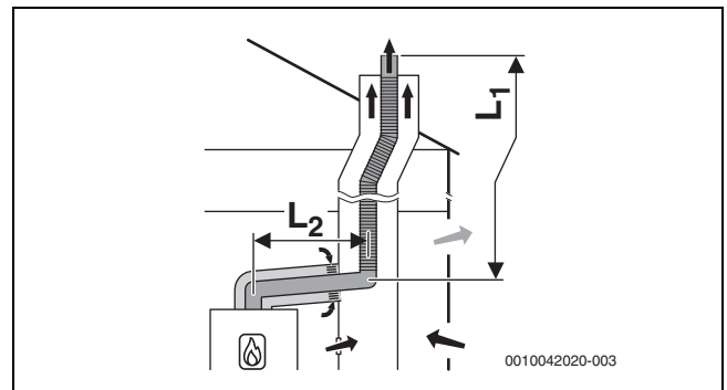
Fig. 17 Ghidarea flexibilă a gazelor arse în puț conform B 53p cu alimentare cu aer dependentă de aerul din încălț prin tronsonul de legătură concentric în încăperea centralei termice; aerisire posterioară în puț
