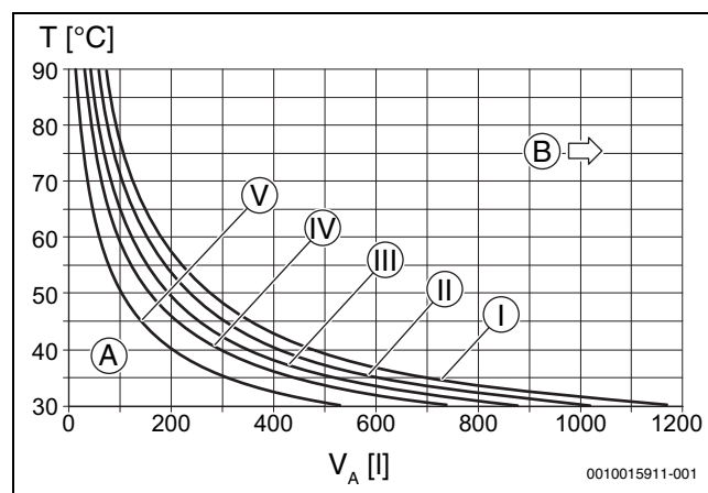
Fig. 29 Curbele caracteristice ale vasului de expansiune
