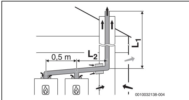
Fig. 27 Cascadă cu 2 aparate: Ghidarea rigidă a gazelor arse în puț conform B 53p cu alimentare cu aer dependentă de aerul din încăperea aparatului și tubulatură pentru gaze arse cu un perete în încăperea centralei termice; aerisire posterioară în puț
