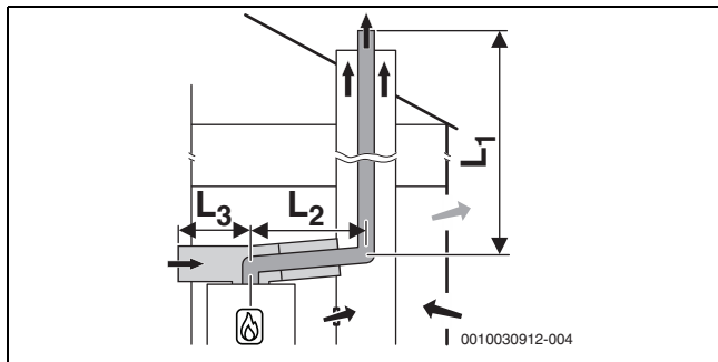
Fig. 11 Ghidarea rigidă a gazelor arse în puț conform C 53x și ghidarea aerului/gazelor arse cu alimentare cu aer separată și evacuare concentrică a gazelor arse în încăperea centralei termice
