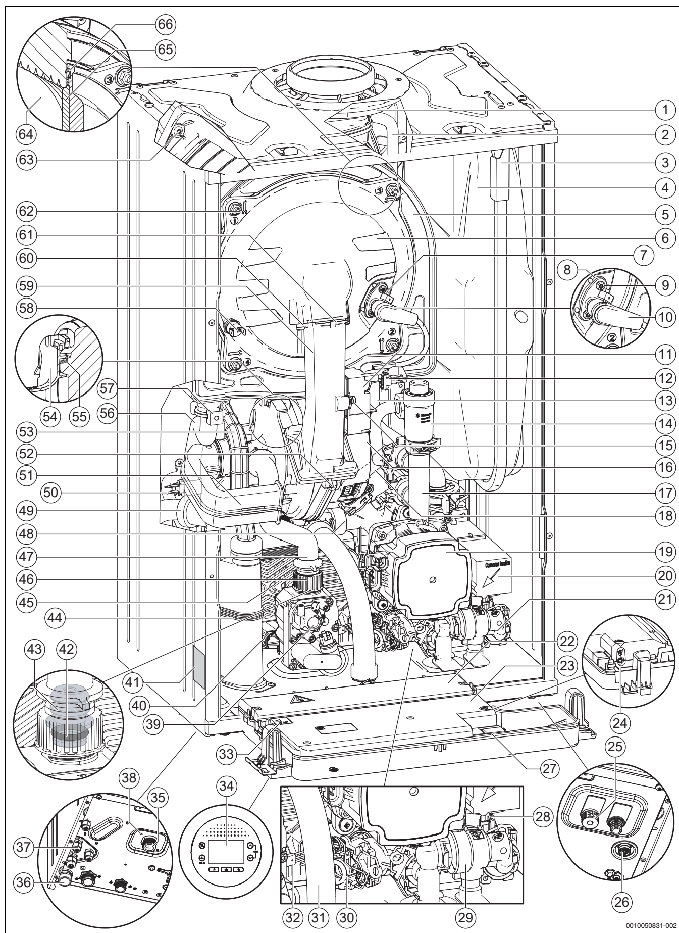
Fig. 3 Structura echipamentului
