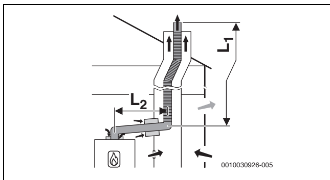
Fig. 19 Ghidarea flexibilă a gazelor arse în puț conform B 53p cu alimentare cu aer dependentă de aerul din încăperea la nivelul aparatului și tubulatură pentru gaze arse cu un perete în încăperea centralei termice; aerisire posterioară în puț
