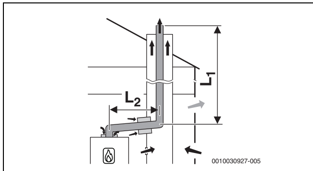
Fig. 18 Ghidarea rigidă a gazelor arse în puț conform B 53p cu alimentare cu aer dependentă de aerul din încăperea la nivelul aparatului și tubulatură pentru gaze arse cu un perete în încăperea centralei termice; aerisire posterioară în puț
